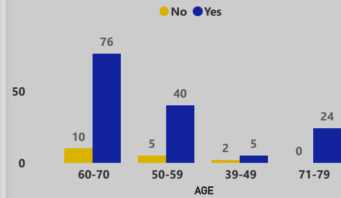
LUNG_CANCER (MALES)
