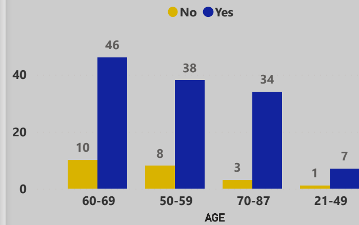
LUNG_CANCER (FEMALES)
